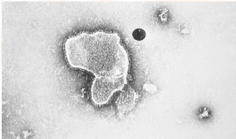
RSウイルスの電子顕微鏡像
